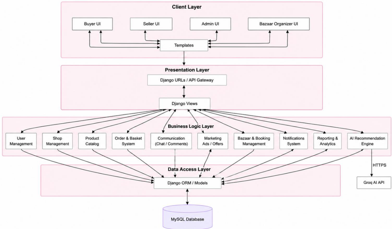
الشكل 82 Component diagram
